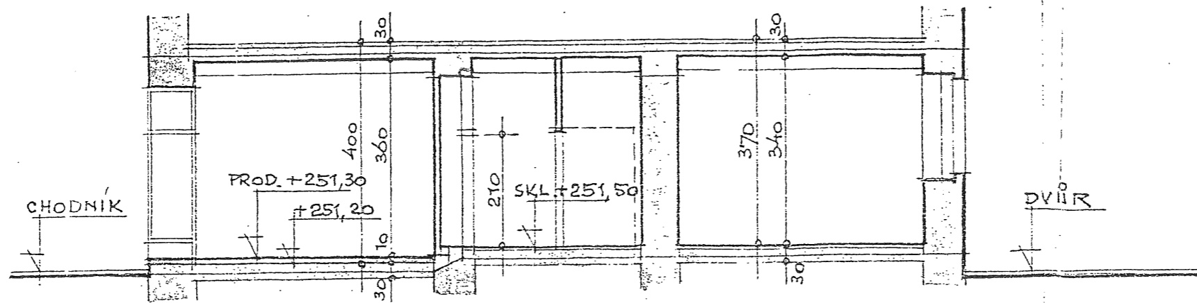
ŘEZ A-A'
